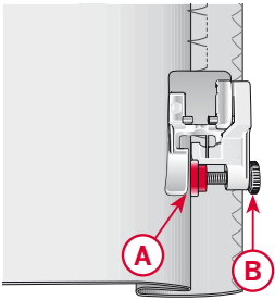
Impostazione per punto per orlo invisibile
