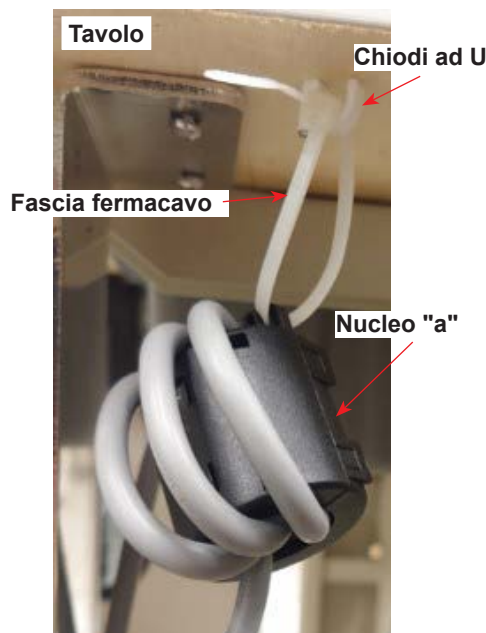
Esempio che mostra il nucleo "a" fissato al tavolo
