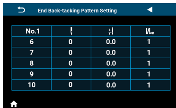
<Schermata di impostazione dell'infittimento personalizzato alla fine della cucitura (2)>
