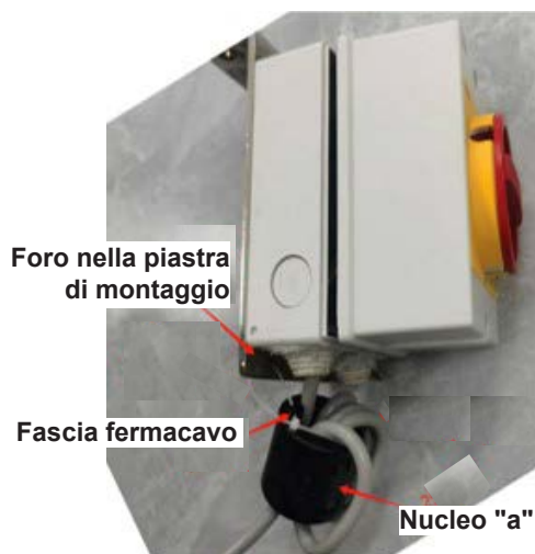
Esempio che mostra il nucleo "a" fissato all'interruttore di alimentazione
