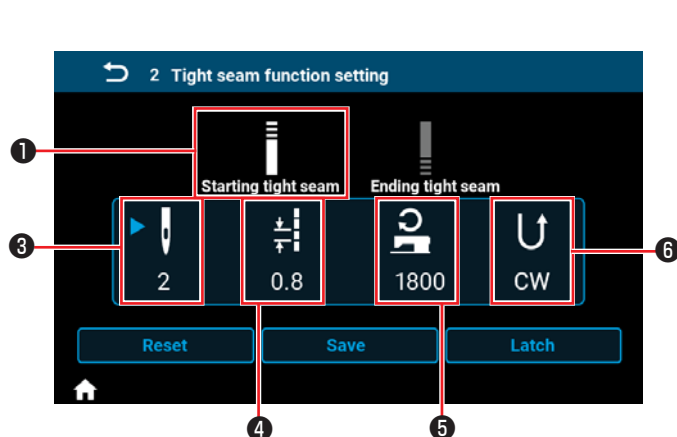
<Schermata di impostazione del punto di infittimento all'inizio della cucitura>
