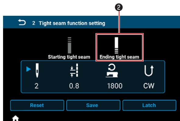
<Schermata di impostazione del punto di infittimento alla fine della cucitura>
