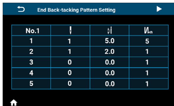
<Schermata di impostazione dell'infittimento personalizzato alla fine della cucitura>
